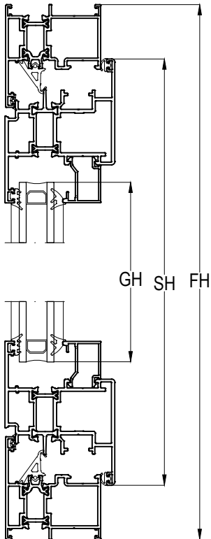
ADAPTÖR PROFİLİ TM55 42 = SH - 66mm
