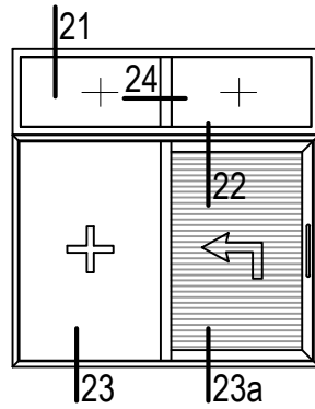
TH55 SİSTEME GEÇİŞ DETAYLARI DETAILS FOR TH55 SYSTEM JOINT
